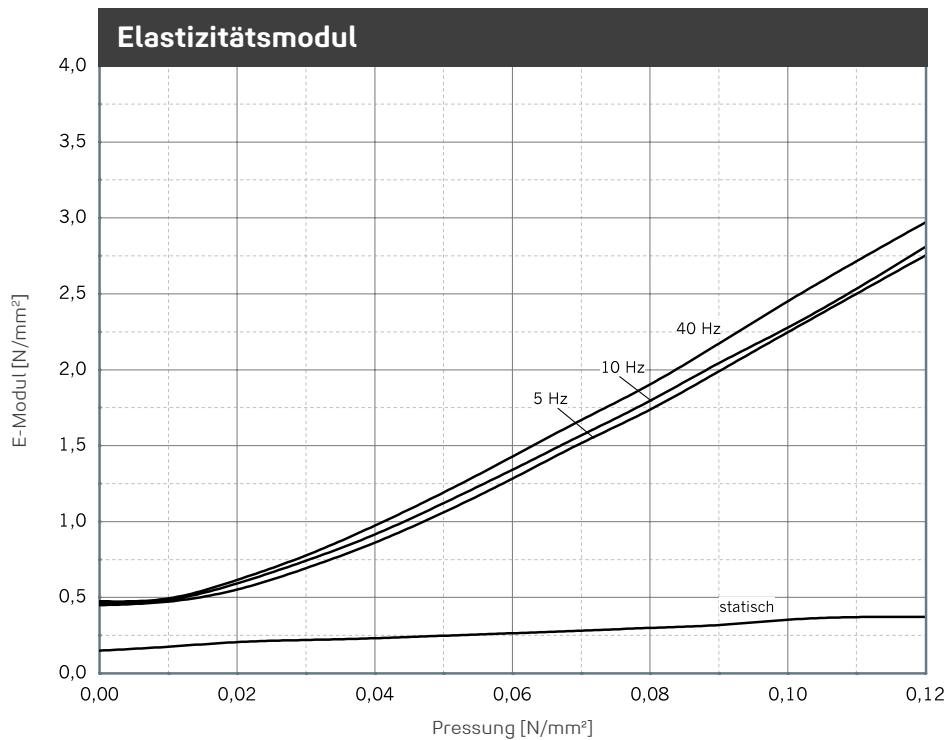
Verlauf des dynamischen E-Moduls bei sinusförmiger Anregung um eine konstante Mittellast, Wegamplitude ± 0,25 mm. Probenabmessung 300 mm x 300 mm x 50 mm; Statischer E-Modul als Tangentenmodul aus der Federkennlinie. Messung in Anlehnung an DIN 53513.
