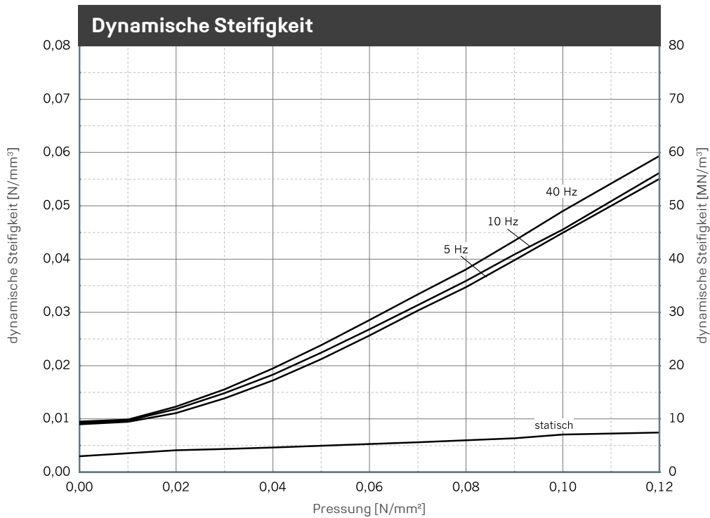
Verlauf der dynamischen Steifigkeit bei sinusförmiger Anregung um eine konstante Mittellast, Wegamplitude ± 0,25 mm. Probenabmessung 300 mm x 300 mm x 50 mm; Statische Steifigkeit als Tangentenmodul aus der Federkennlinie. Messung in Anlehnung an DIN 53513.
